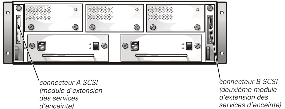
Figure 2-3. Panneau arrière
